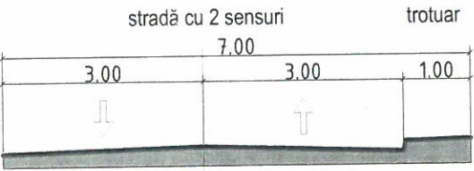
PROFIL TRANSVERSALA A-A
