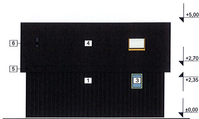
FAȚADĂ FRONTALĂ
