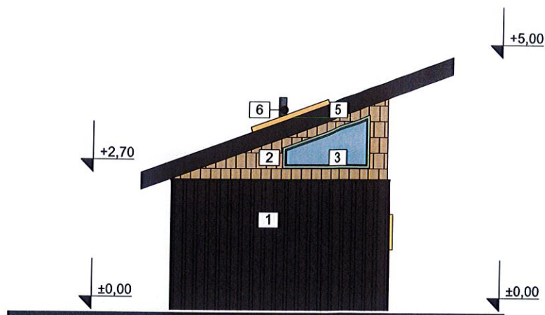
FAȚADĂ LATERALĂ STÂNGĂ
